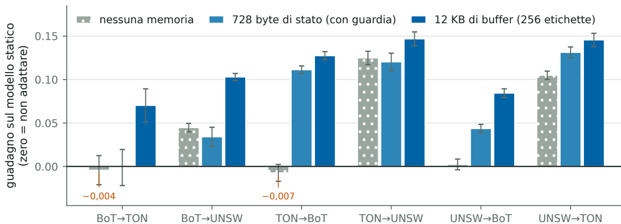
(c) cosa costa la memoria che il dispositivo non ha — rapporto 1:50, 10 seed
