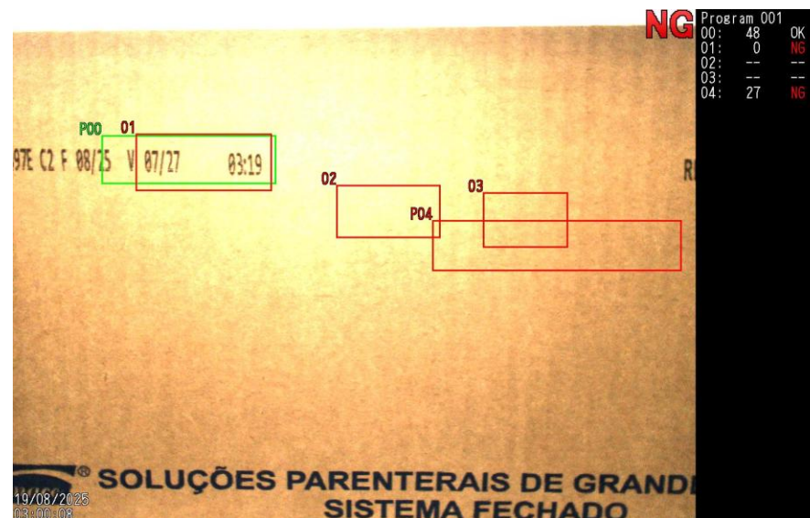
CAM 4 – Impressão Fora da Posição
