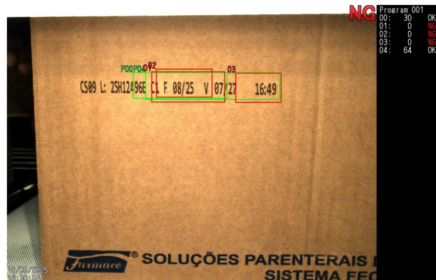
CAM 4 – Impressão Fora de Posição (Esquerda)
