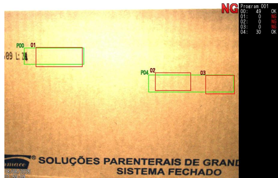
CAM 4 – Impressão Incompleta
