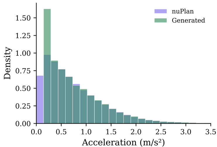
(d) IDM Acceleration
