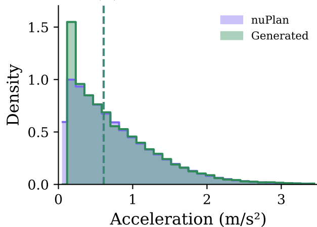
(d) IDM Acceleration
