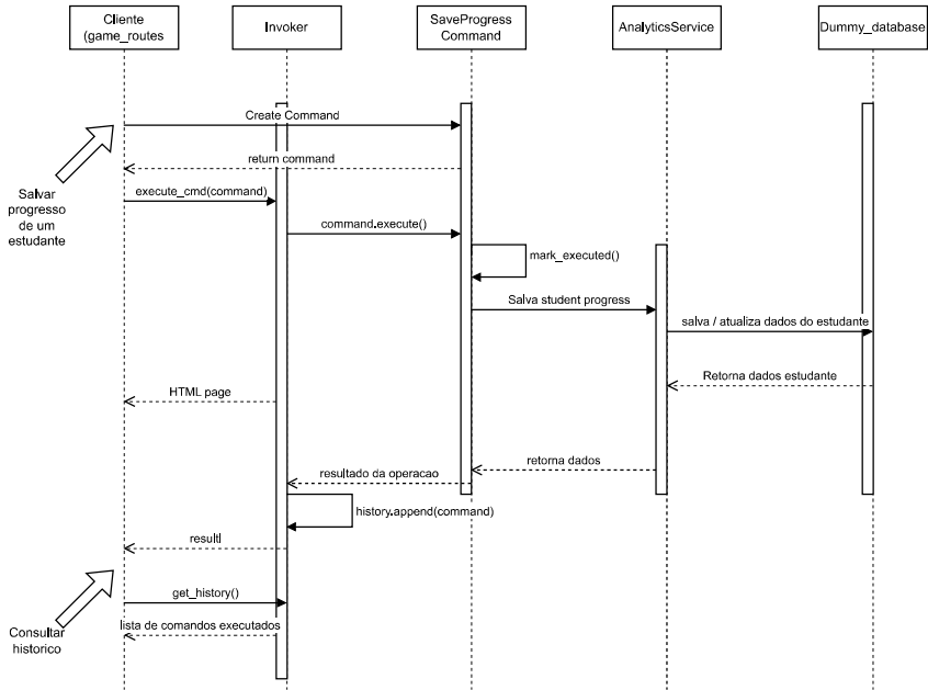
Diagrama de sequencia de SaveProgressStudent com Padrao Command e consulta de historico ao final
