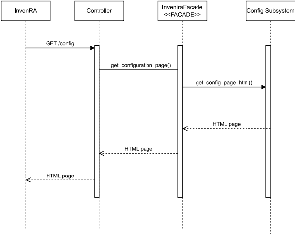
Diagrama de sequencia da operacao Get /config com facade e subsystem Config
