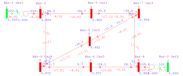
Figura 2. Simulação do caso base do STB-9 no ANAREDE.
