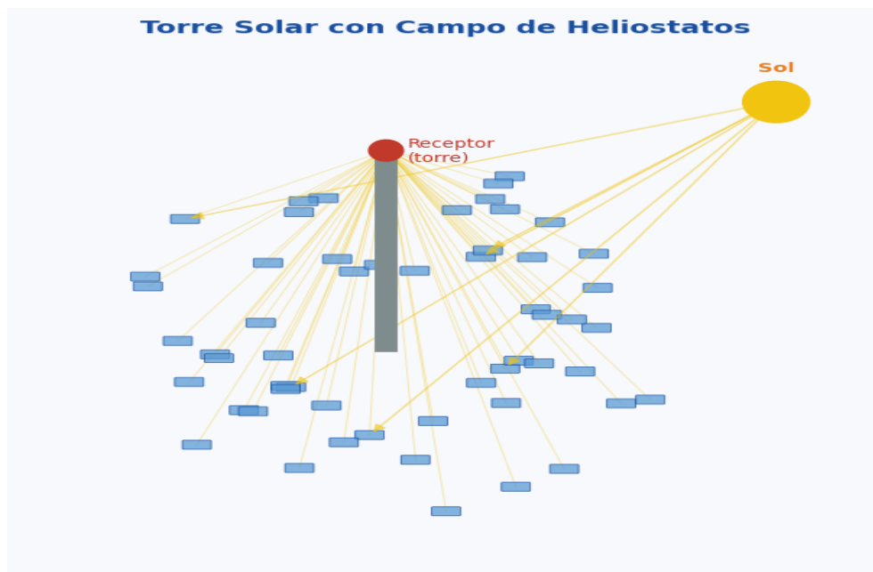
Fig. 5 — Esquema de Torre Solar con Campo de Heliostatos. Cada heliostato sigue al Sol de forma independiente y refleja la luz hacia el receptor en la torre central.
