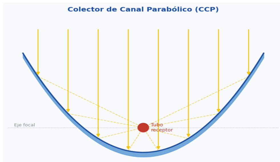
Fig. 1 — Sección transversal del Colector de Canal Parabólico (CCP). Los rayos solares paralelos son reflejados hacia el tubo receptor ubicado en el foco.
