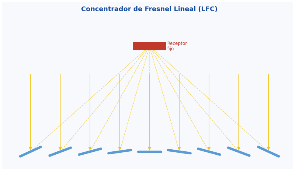
Fig. 2 — Vista lateral del Concentrador de Fresnel Lineal. Cada espejo plano refleja la radiación hacia el receptor fijo en la parte superior.
