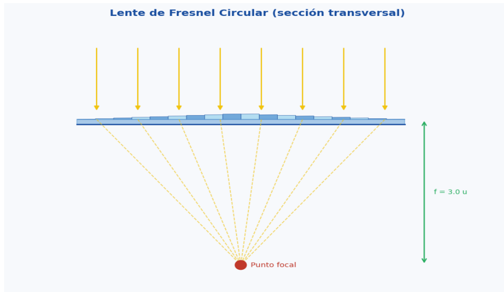
Fig. 6 — Sección transversal de la Lente de Fresnel Circular. El perfil escalonado refracta los rayos paralelos hacia un único punto focal.
