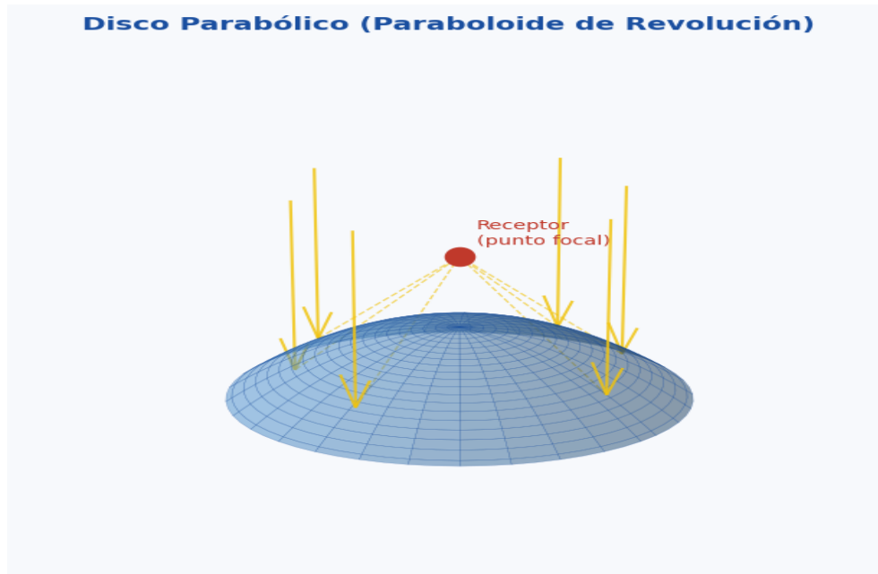
Fig. 4 — Vista 3D del Disco Parabólico. Los rayos solares se reflejan desde toda la superficie del paraboloide hacia el receptor ubicado en el punto focal.
