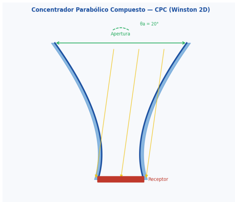
Fig. 3 — Sección transversal del CPC de Winston. Las dos parábolas dirigen toda la radiación dentro del ángulo de aceptación ( \theta_a ) hacia el receptor.
