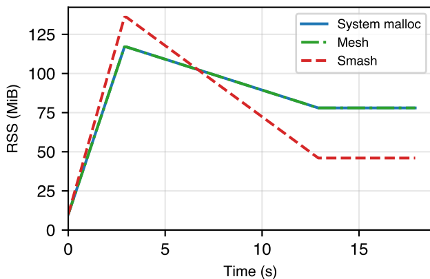
Redis-ext (macOS)
