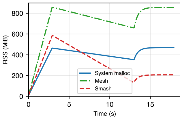
Redis (Linux)
