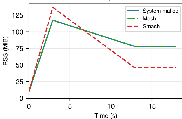
Redis-ext (macOS)
