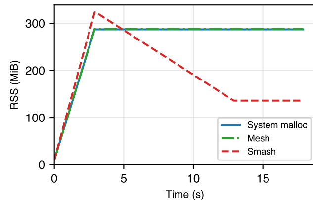
SQLite (macOS)
