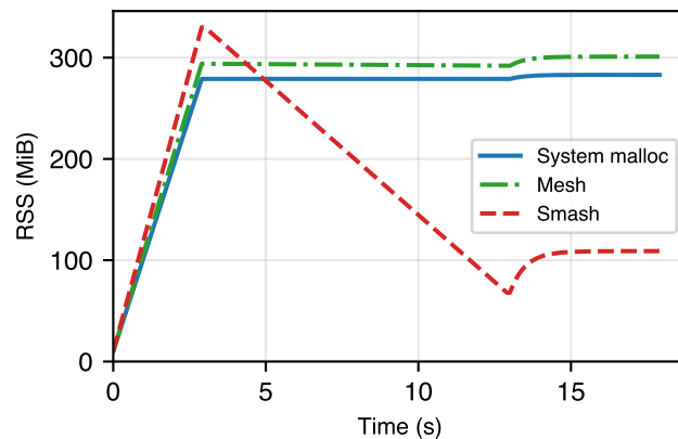
Redis-ext (Linux)
