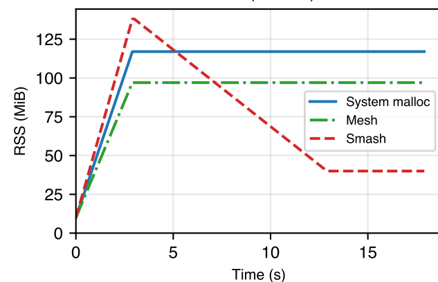
Redis (macOS)
