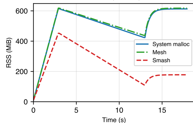
Redis (macOS)
