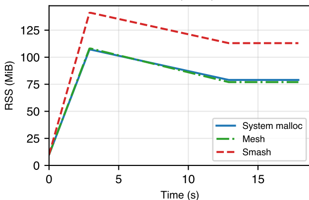
RocksDB (macOS)
