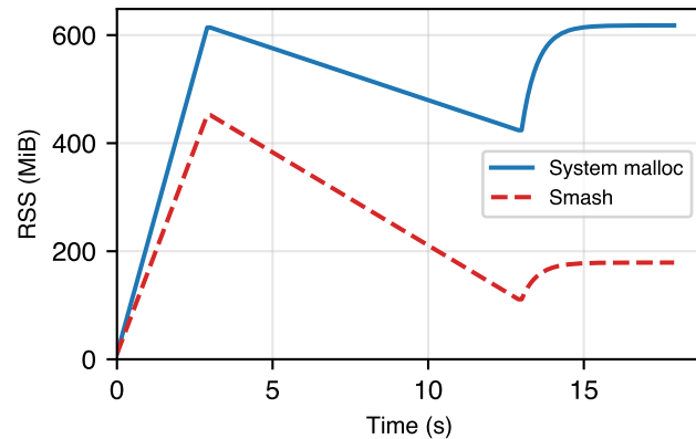
SQLite (macOS)
