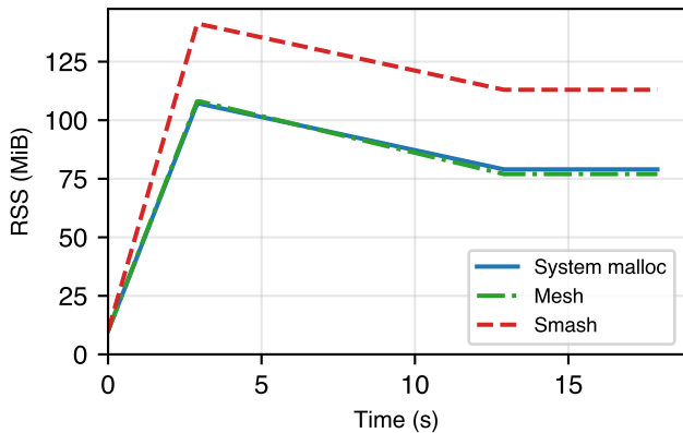
Redis (Linux)
