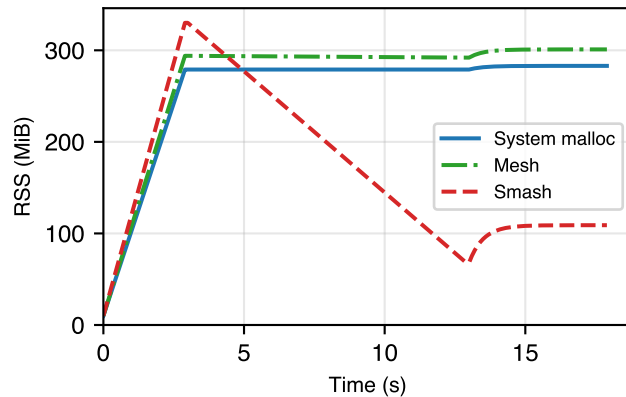
Redis-ext (Linux)
