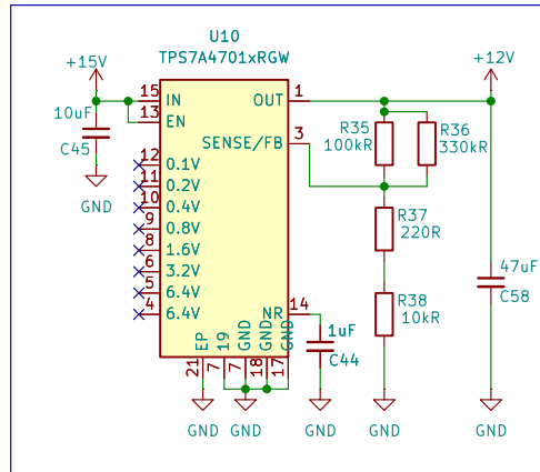
+15V -> +12V
