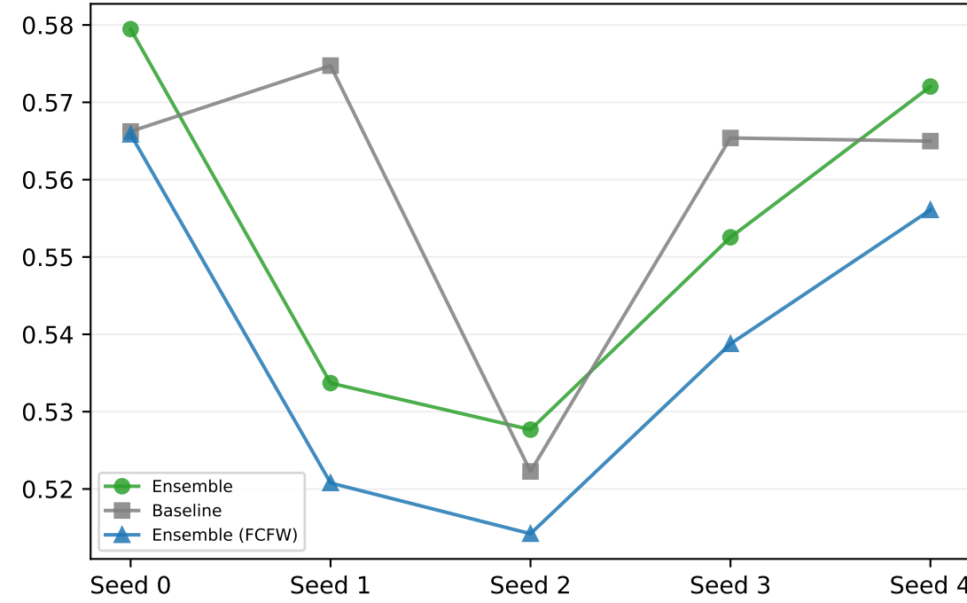
tvd_exact
