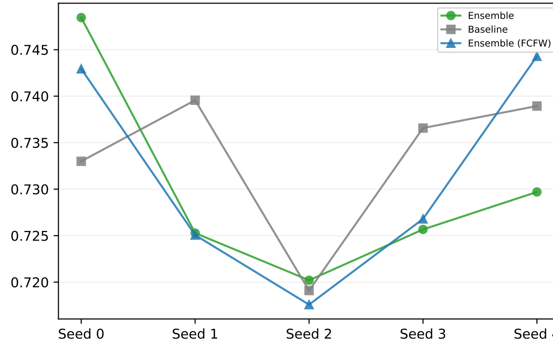
kl_exact
