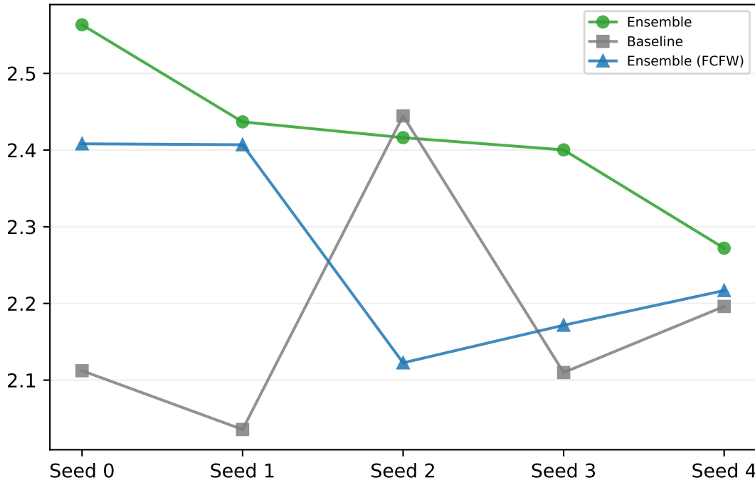
kl
