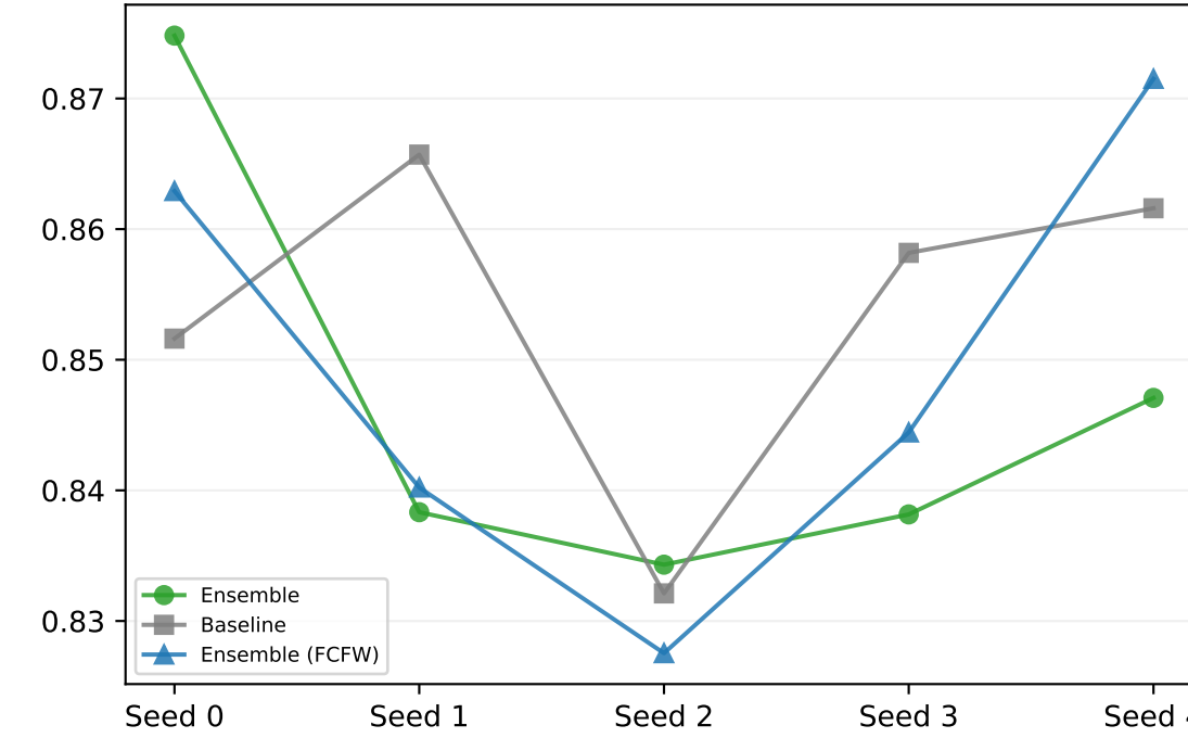
tvd
