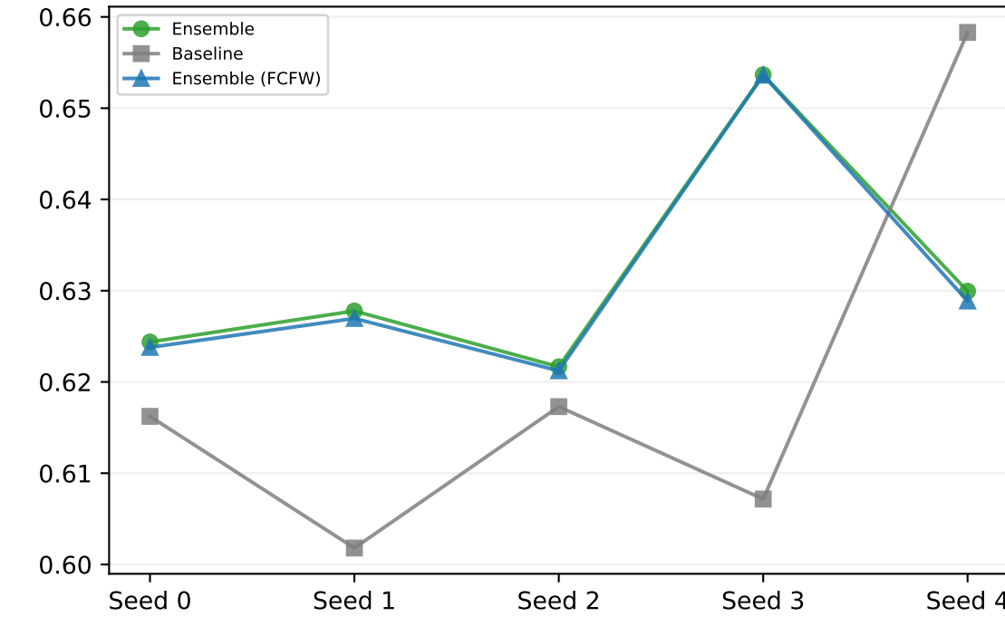
tvd_exact
