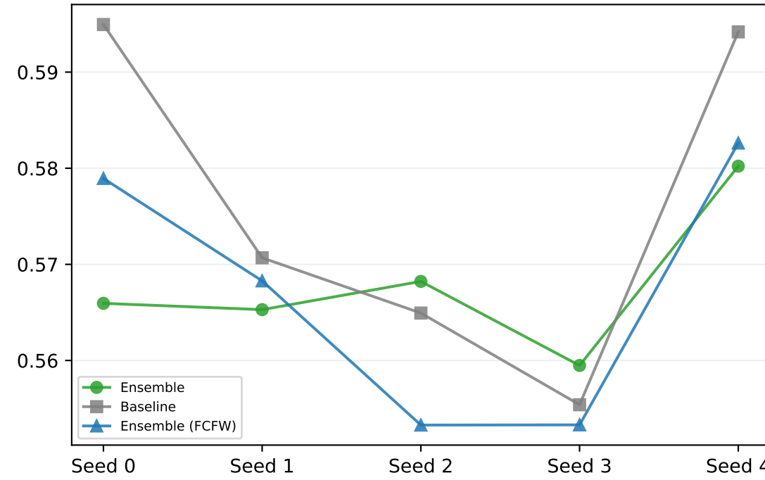
kl_exact
