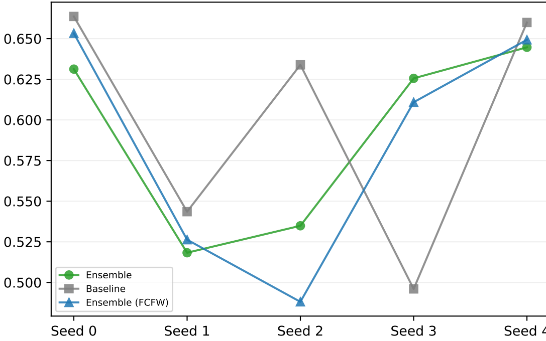
tvd
