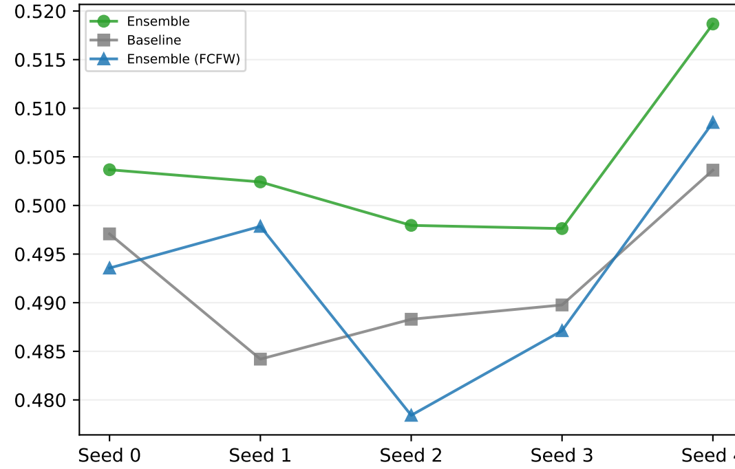
kl_exact
