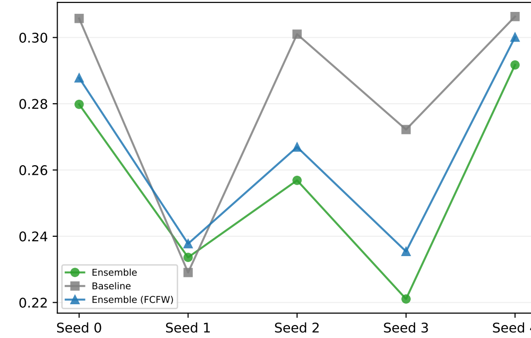
tv_d
