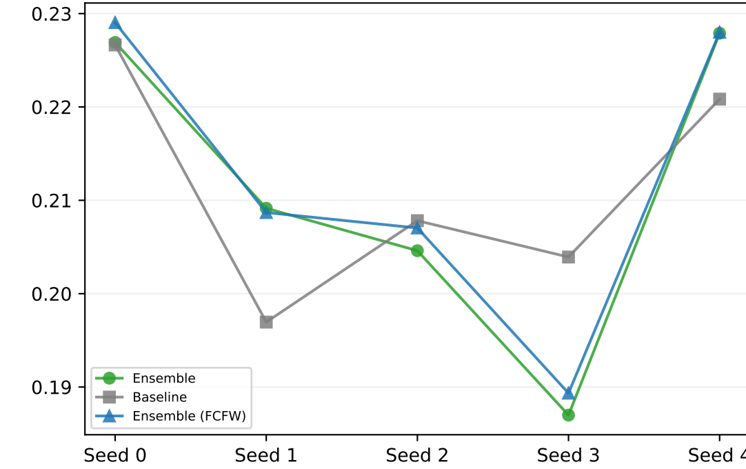
tv_d_exact
