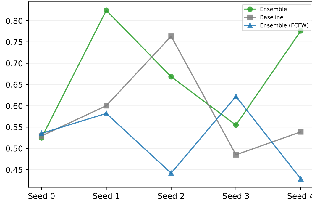
kl
