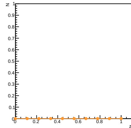
Perfil de densidade N(100)
