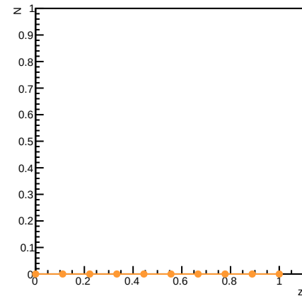
Perfil de densidade N(10)
