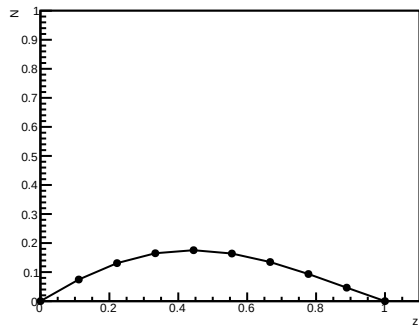
Perfil de densidade N(15)
