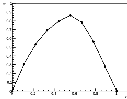
Perfil de densidade N(3)
