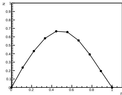
Perfil de densidade N(5)
