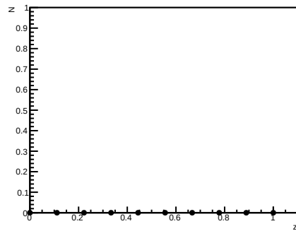
Perfil de densidade N(100)
