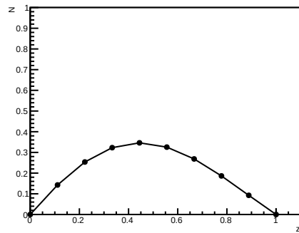
Perfil de densidade N(10)
