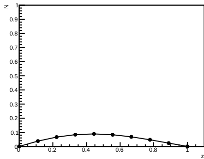
Perfil de densidade N(20)
