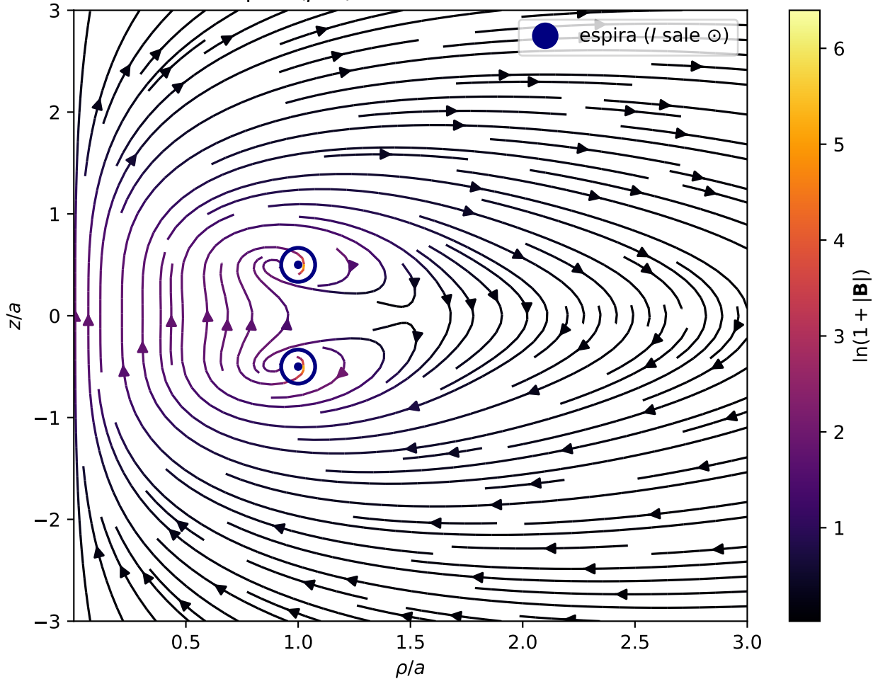
Campo \mathbf{B}(\rho, z) — Bobina de Helmholtz
