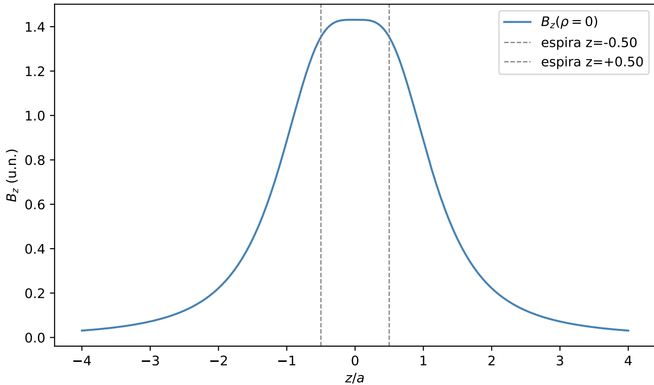
B_z en el eje — Bobina de Helmholtz ( d = a )
