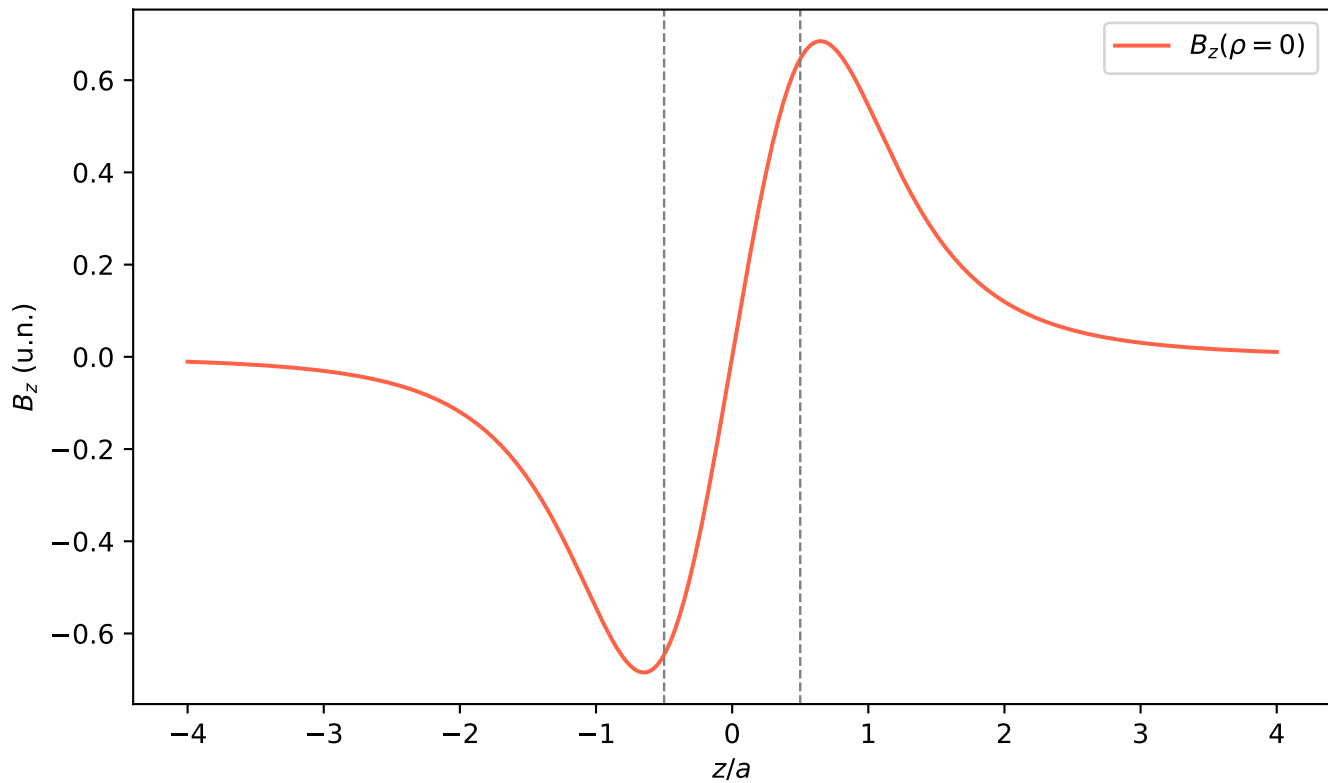
B_z en el eje — Anti-Helmholtz ( d = a )
