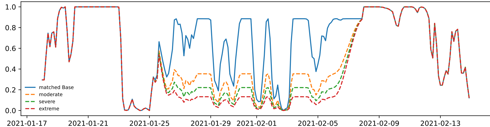
DE0 0 0 offwind-dc
