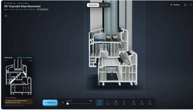
X = 230: A yarığı kesiliyor.
