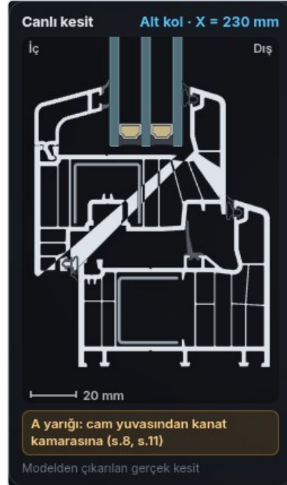
Canlı kesit penceresi (yakın).
