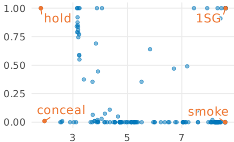
Sino-Tibetan
