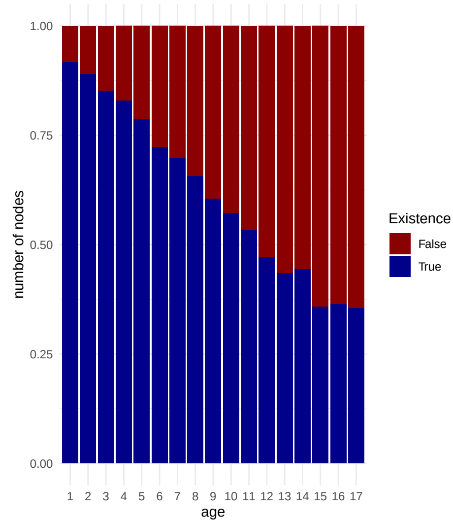
Hipstr
