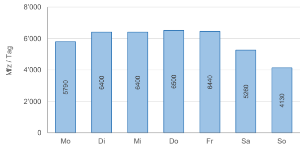
Durchschnittliche Wochenganglinie (DTV gerundet)
