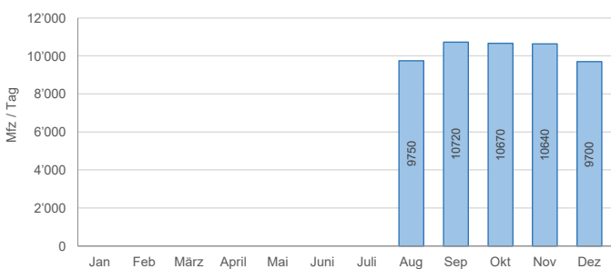
Durchschnittliche Jahresganglinie (DTV gerundet)
