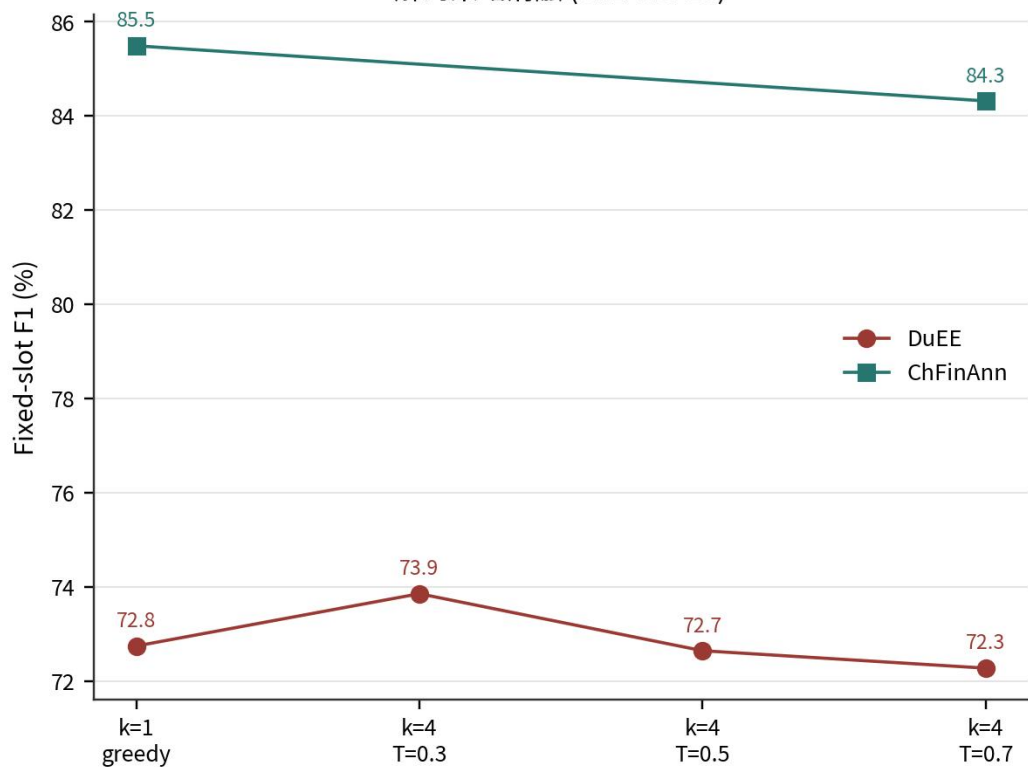
解码策略消融 (vLLM BF16)
