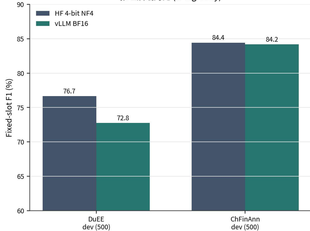
推理后端对比 (k=1 greedy)
