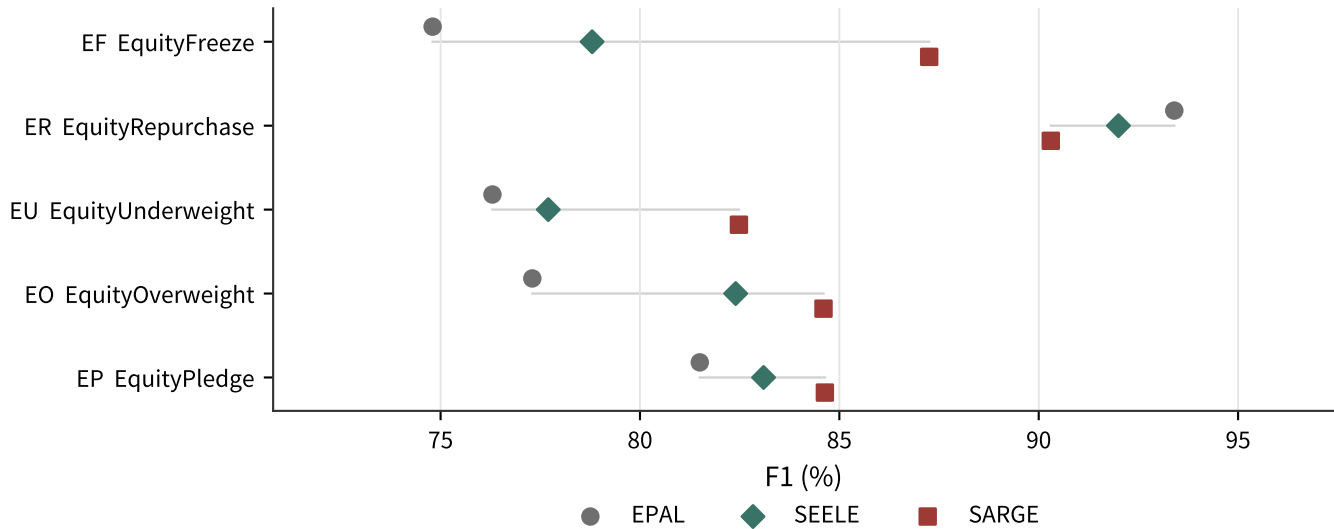
ChFinAnn 分事件类型 F1
