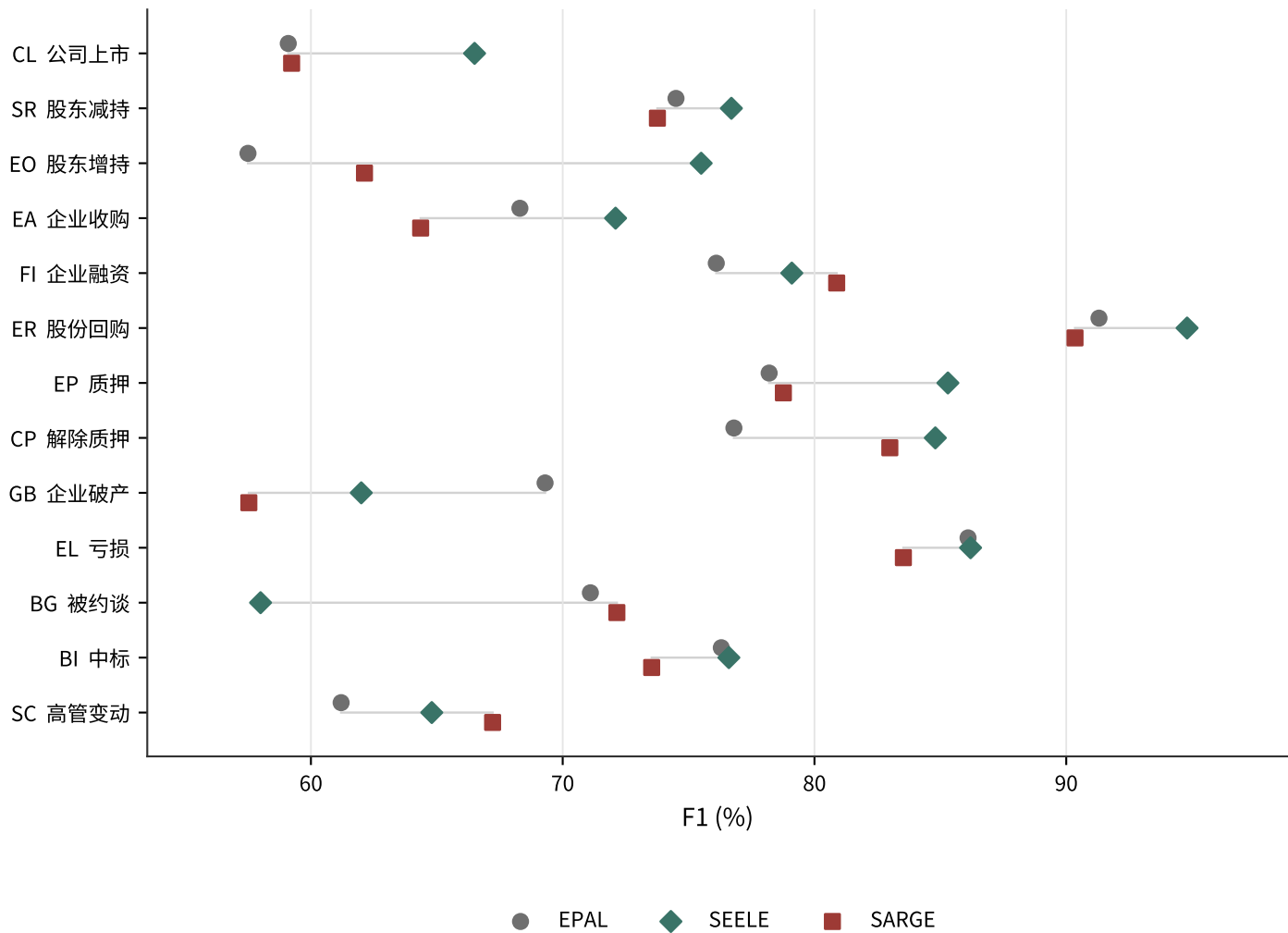
DuEE-Fin 分事件类型 F1
