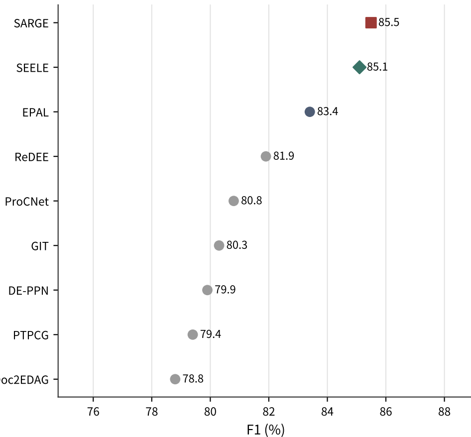
ChFinAnn-Doc2EDAG
