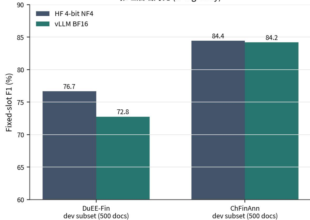
推理后端对比 (k=1 greedy)
