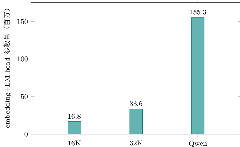
词汇量 vs 参数 (hidden=512, 不共享权重)
