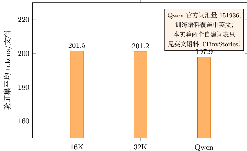
词汇量 vs 序列长度 (TinyStories 验证集)
