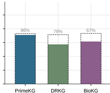
Llama-3.3-70B
