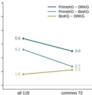
Llama-3.3-70B
