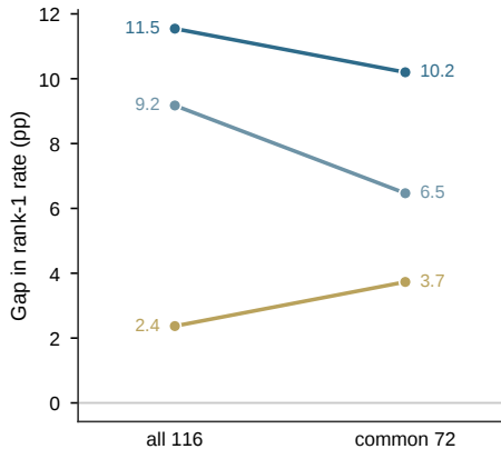
GPT-4.1-mini
