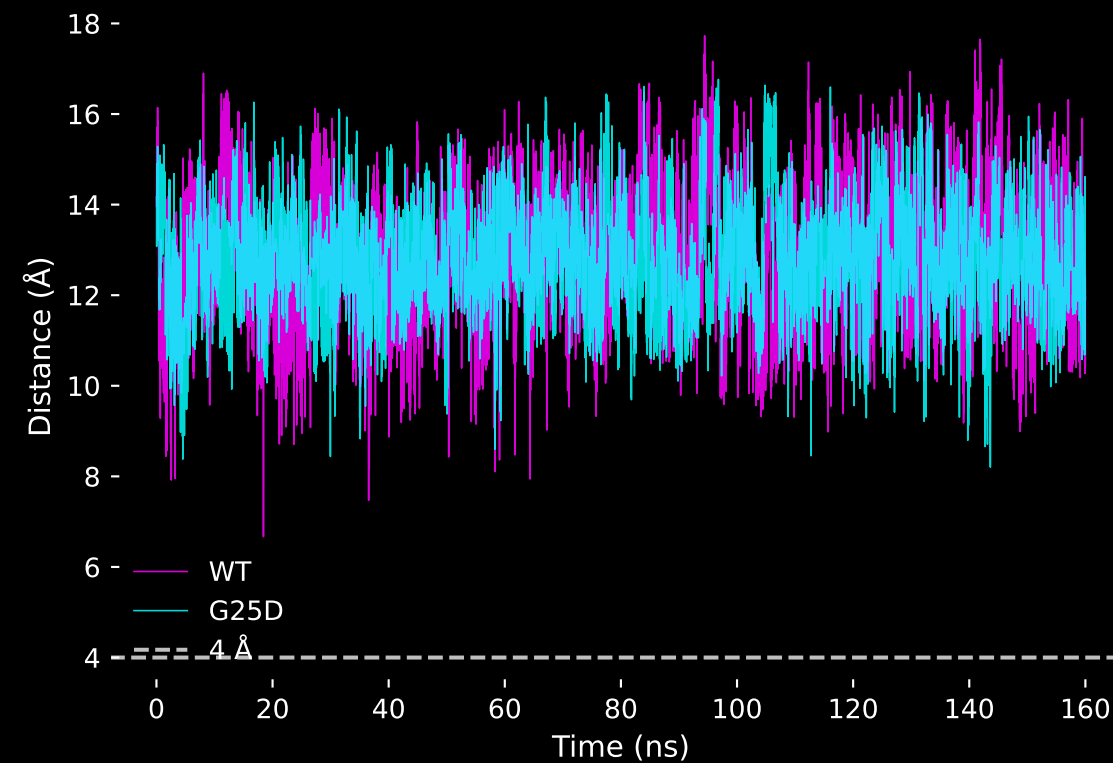
(D) D23-K28 Salt Bridge
