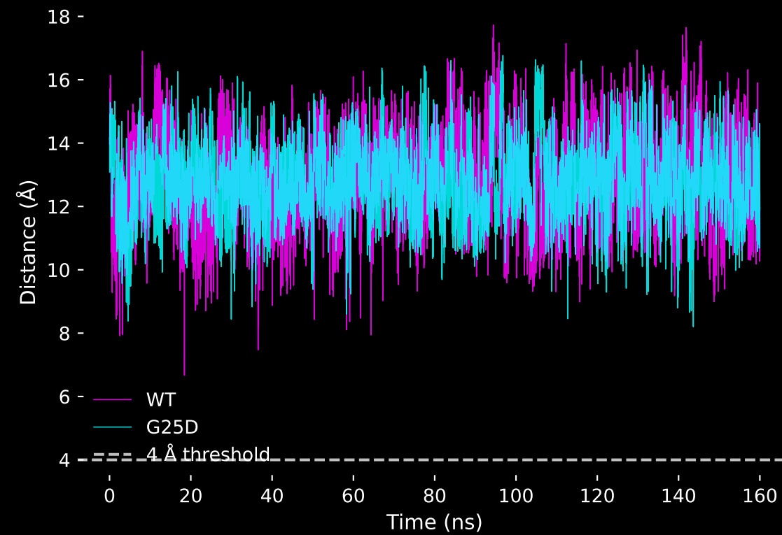
(D) D23-K28 Salt Bridge Distance
