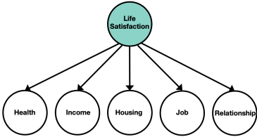
Top-Down (Dispositional)
