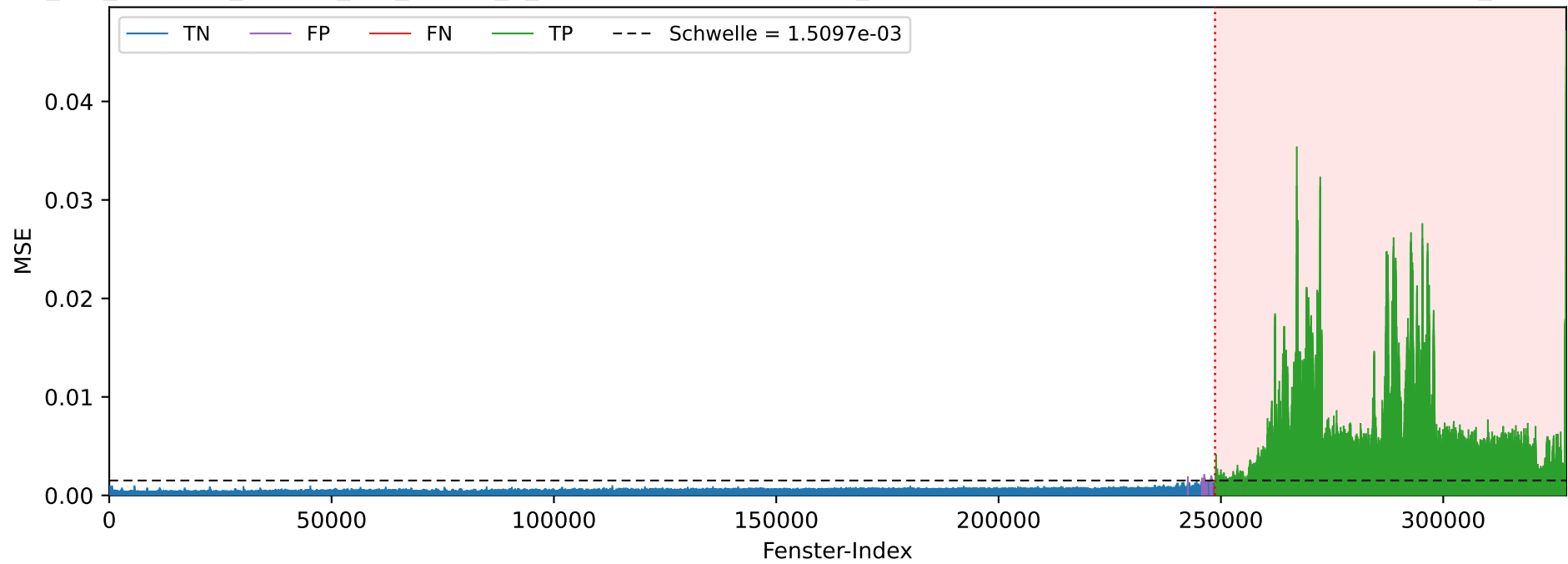
model_lfW_eID1009_flip.csv_run_fedrep_6_clients - FULL MSE (p99_99, Schwelle auf Normalfenstern) - Datei: lfW_eID1009_flip.csv
