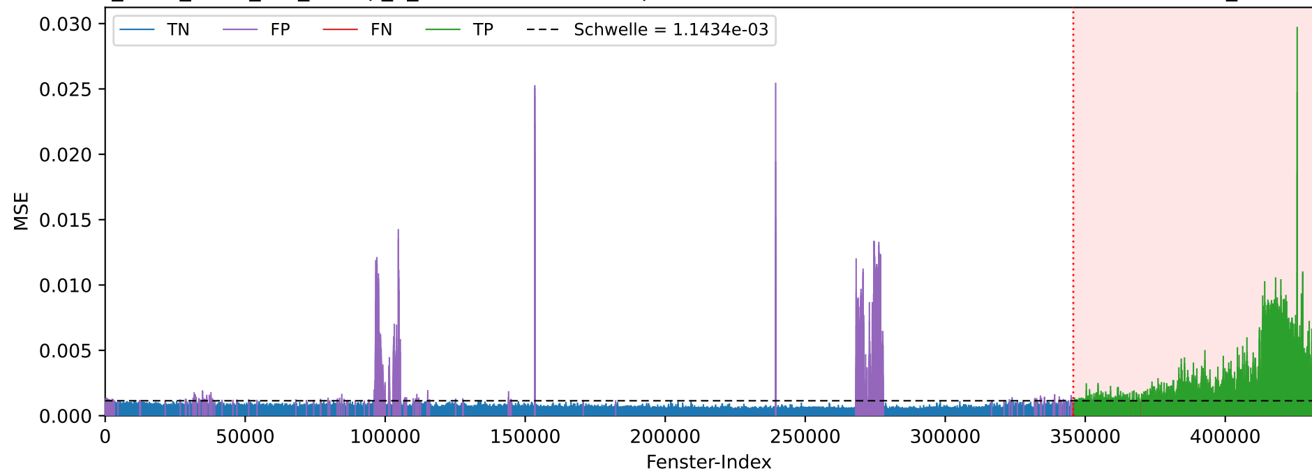
model_ES35_1.csv_run_fedrep_6_clients - FULL MSE (p99, Schwelle auf Normalfenstern) - Datei: Paulhorn_eID1006.csv
