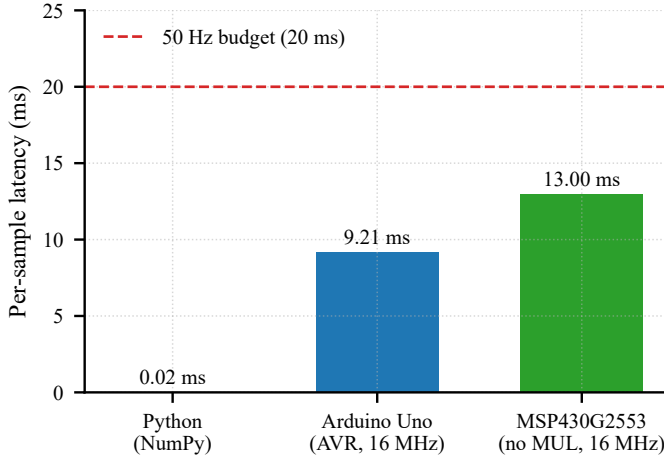
Şekil 7. Üç referans platformda örnek-başına çıkarım gecikmesi. Kırmızı kesikli çizgi, 50 Hz örnekleme hızının getirdiği 20 ms bütçeyi gösterir. Her iki MCU hedefi de bütçenin belirgin biçimde altında çalışır.
