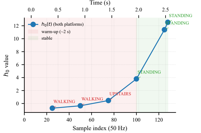
Şekil 8. Tek bir 2,56 s pencerede (50 Hz, STANDING gerçek etiketi) gizli durum bileşeni h_0 ve üretilen sınıf etiketi. Arduino ve MSP430 aynı yörüngeleri üretir. Yaklaşık 2 s geçmiş birikene kadar sınıf etiketi kararsızdır.
