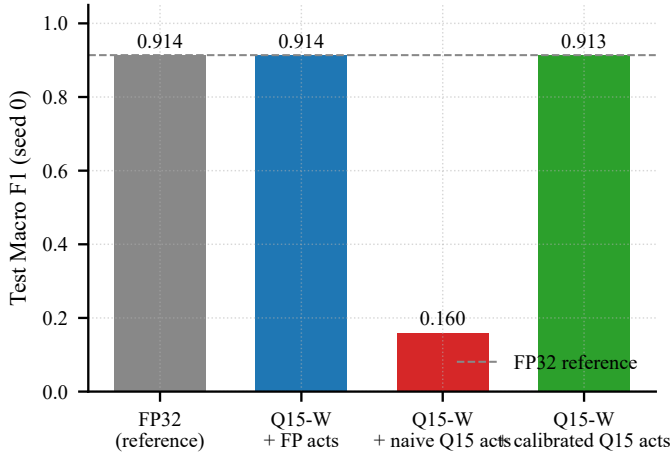
Şekil 5. Seed-0 modelinde nicelendirme kipleri. Yalnızca ağırlık Q15 kayıpsızdır; saf Q15 aktivasyonları modeli çökertir; kalibre edilmiş Q15 aktivasyonları referansı yuvarlama gürlütüsü içinde geri kazanır.
