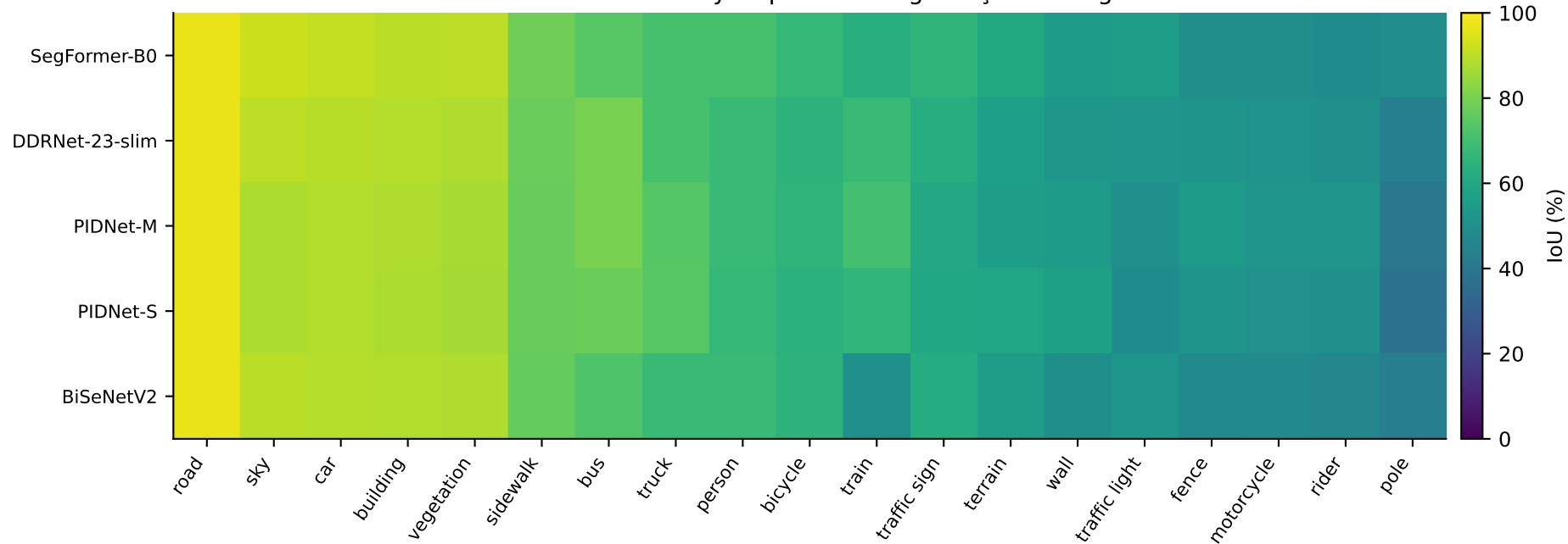
Sınıf bazlı IoU · Cityscapes val · dağıtım çözünürlüğü
