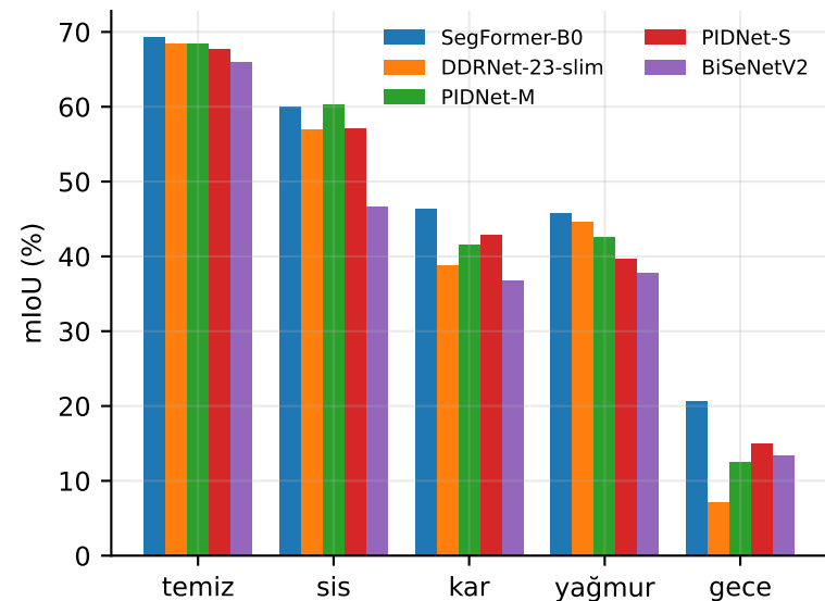
Doğruluk · koşul başına
