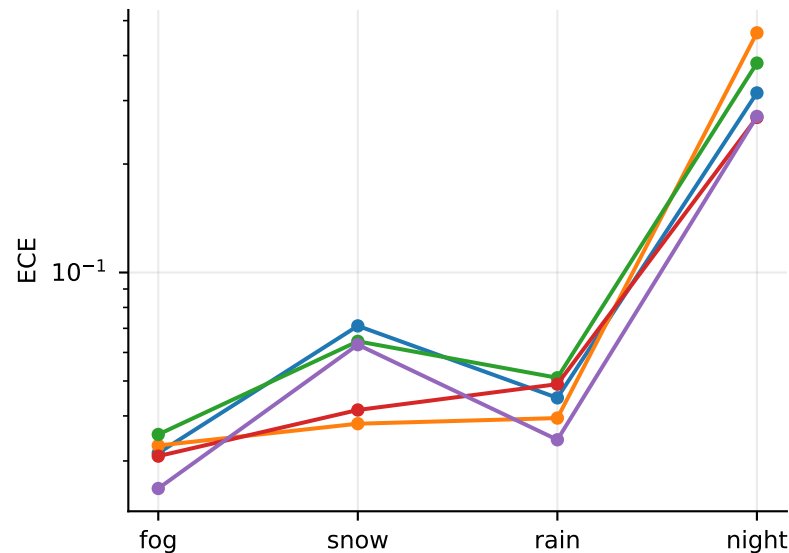
Kalibrasyon · gecede 9-14x bozuluyor
