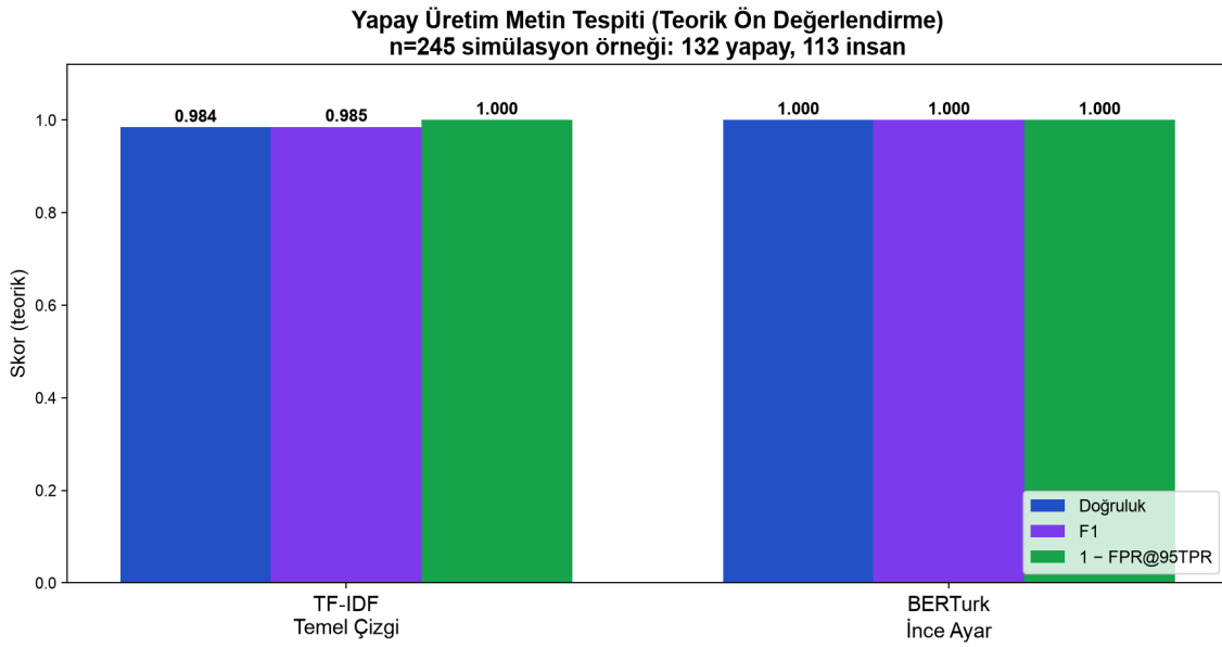
Şekil 2. Yapay Üretim Metin Tespiti — Model Karşılaştırması (n=245: 132 yapay, 113 insan)
