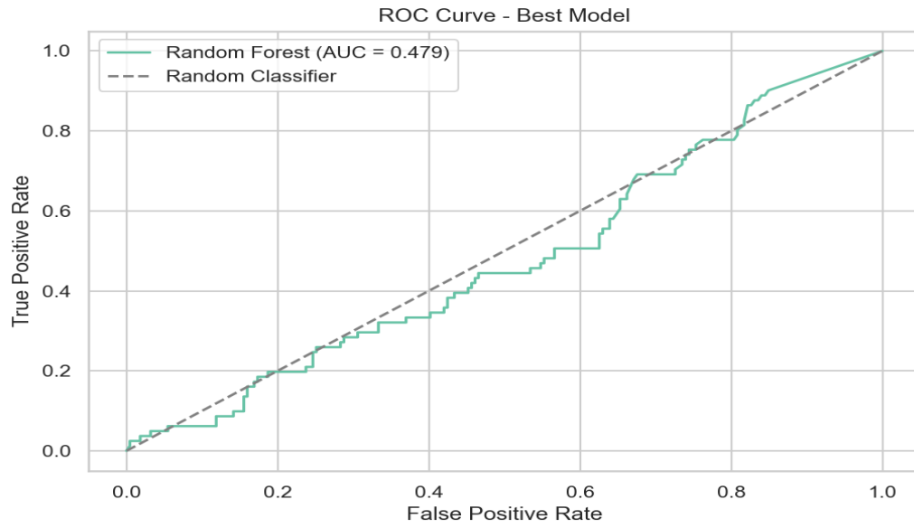
Şekil 4: ROC eğrisi
