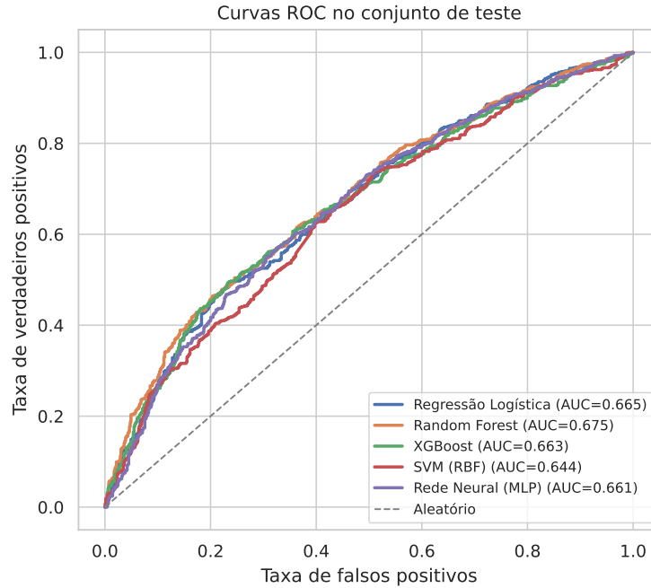
Figura 3: Curvas ROC no conjunto de teste.
