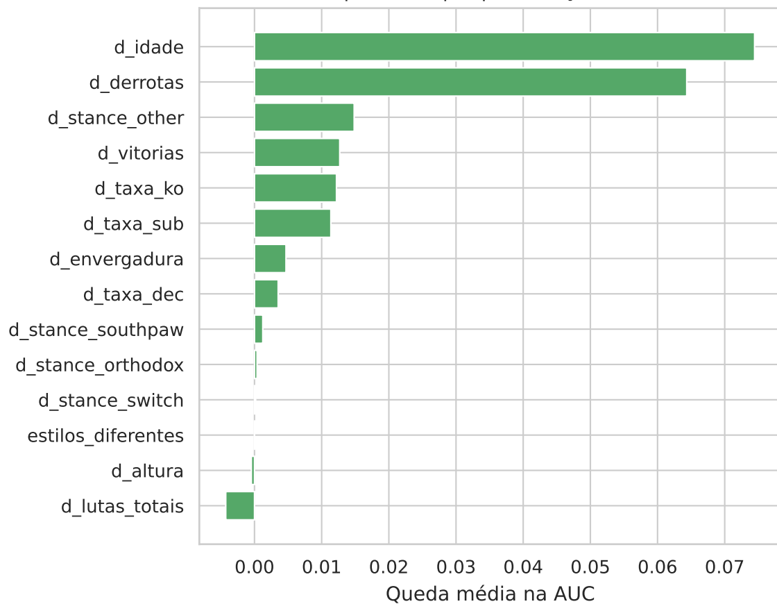
Importância por permutação (AUC)
