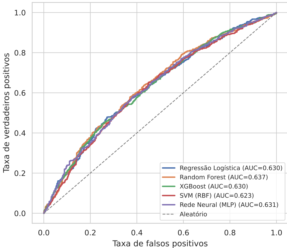
Curvas ROC no conjunto de teste
