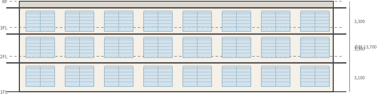
南立面図
