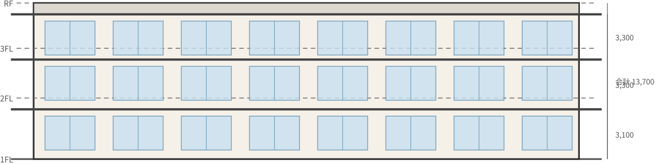
北立面図
