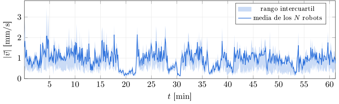
Figura 21: Rapidez de los robots en función del tiempo.
