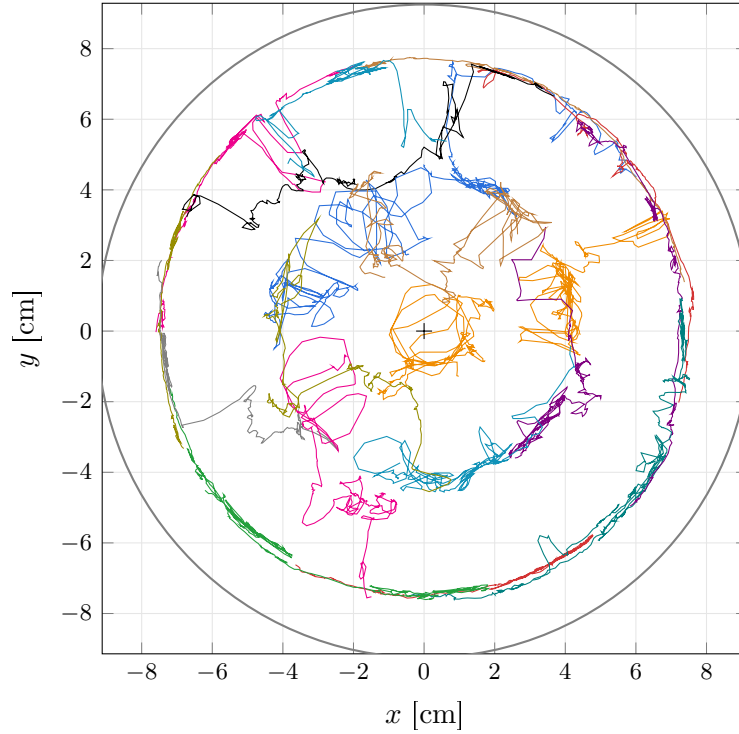
Figura 23: Trayectorias de los 22 robots (escena real, video espejado corregido; origen en el centro del recinto, y hacia arriba; círculo gris: pared interior), primeros 5 minutos reales.
