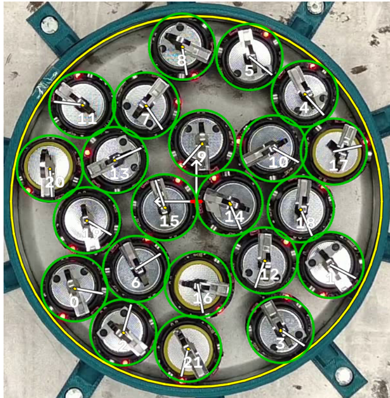
Figura 20: Cuadro de ejemplo con identificador, vector velocidad (amarillo, largo = desplazamiento en 7,5 cuadros) y orientación (aguja blanca). Círculo verde: posición observada; naranja: estimada. Imagen tal como la graba la cámara (espejada); flecha y aguja dibujadas sobre ella.
