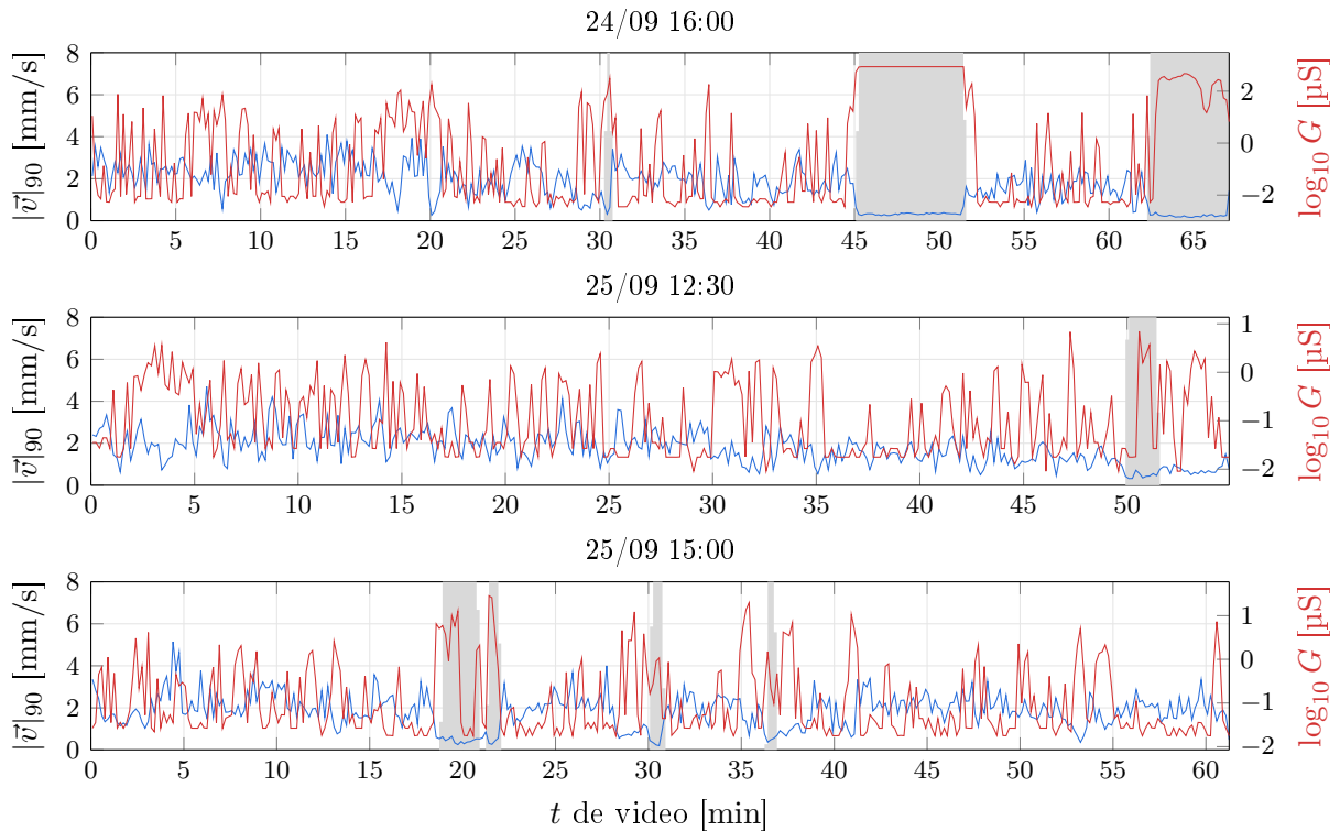
Figura 9: Movilidad de los robots (percentil 90 de la rapidez, azul; atascos sombreados) y conductancia del sensor de presión G = 1/R (rojo, escala logarítmica, medianas de 10s), con el registro alineado al fin del pulso LED de sincronización (tabla 9).
