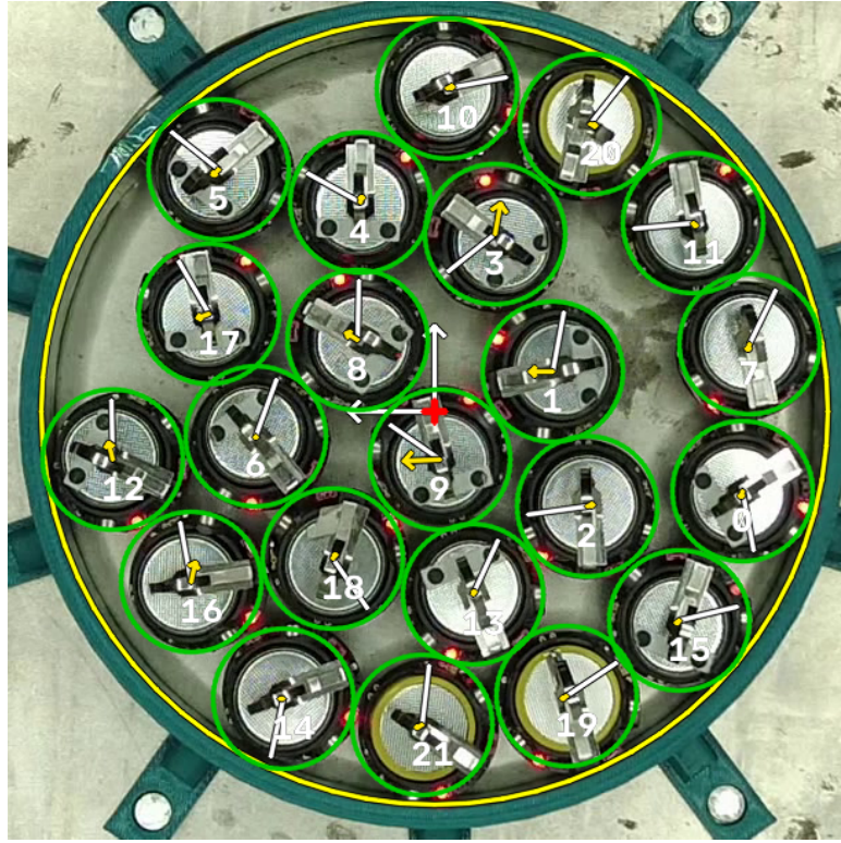
Figura 10: Cuadro de ejemplo con identificador, vector velocidad (amarillo, largo = desplazamiento en 7,5 cuadros) y orientación (aguja blanca). Círculo verde: posición observada; naranja: estimada. Imagen tal como la graba la cámara (espejada); flecha y aguja dibujadas sobre ella.
