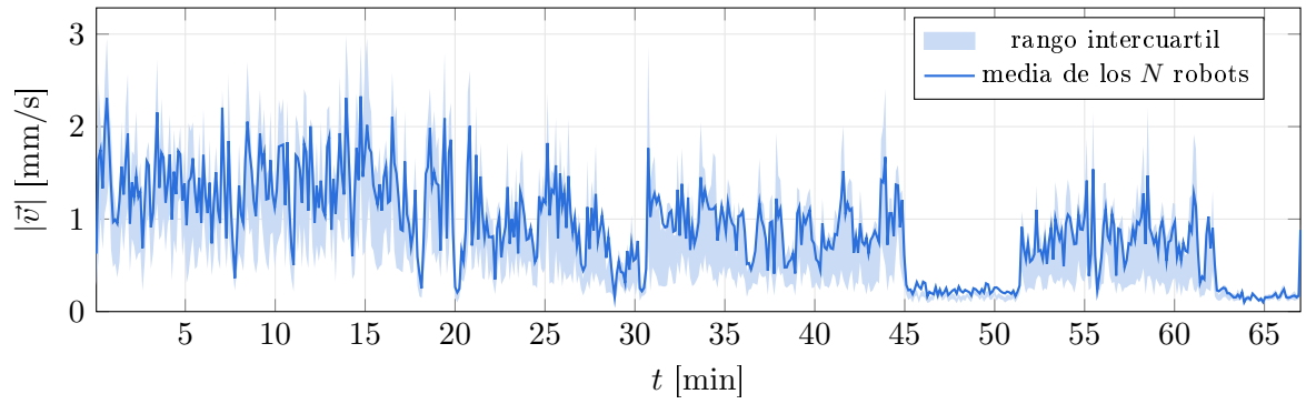
Figura 11: Rapidez de los robots en función del tiempo.
