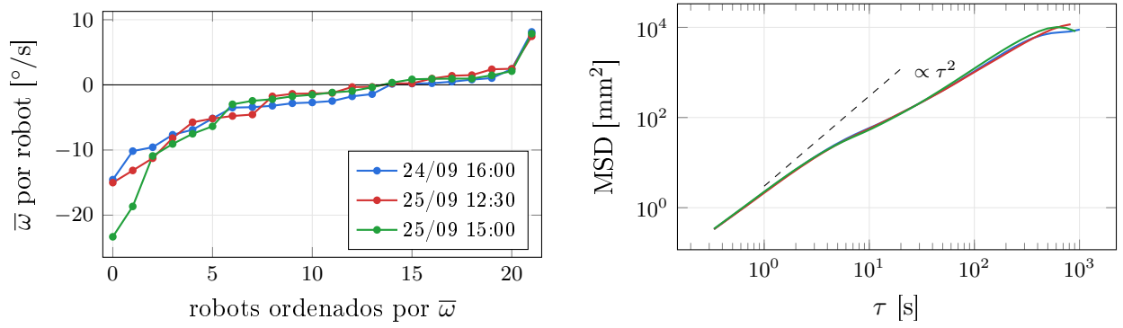
Figura 5: Izq.: velocidad angular media de cada robot, ordenada (cada punto es un robot). Der.: desplazamiento cuadrático medio \text{MSD}(\tau) = \langle |\vec{r}(t+\tau) - \vec{r}(t)|^2 \rangle ; la recta de referencia indica movimiento balístico.
