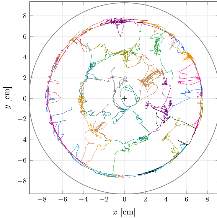
Figura 18: Trayectorias de los 22 robots (escena real, video espejado corregido; origen en el centro del recinto, y hacia arriba; círculo gris: pared interior), primeros 5 minutos reales.
