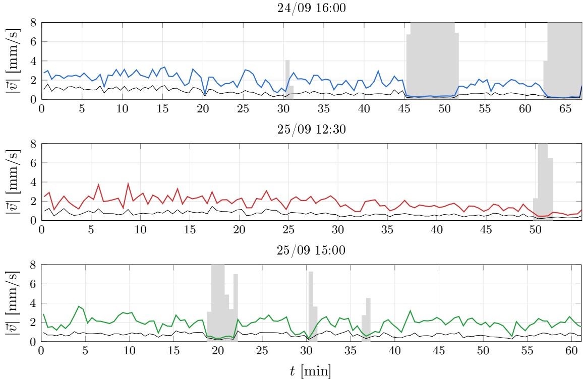
Figura 3: Evolución de la rapidez en ventanas de 30 s: percentil 90 entre robots (color) y mediana (negro). Sombreado: atascos (percentil 90 suavizado < 0,52 mm/s durante al menos 20 s).
