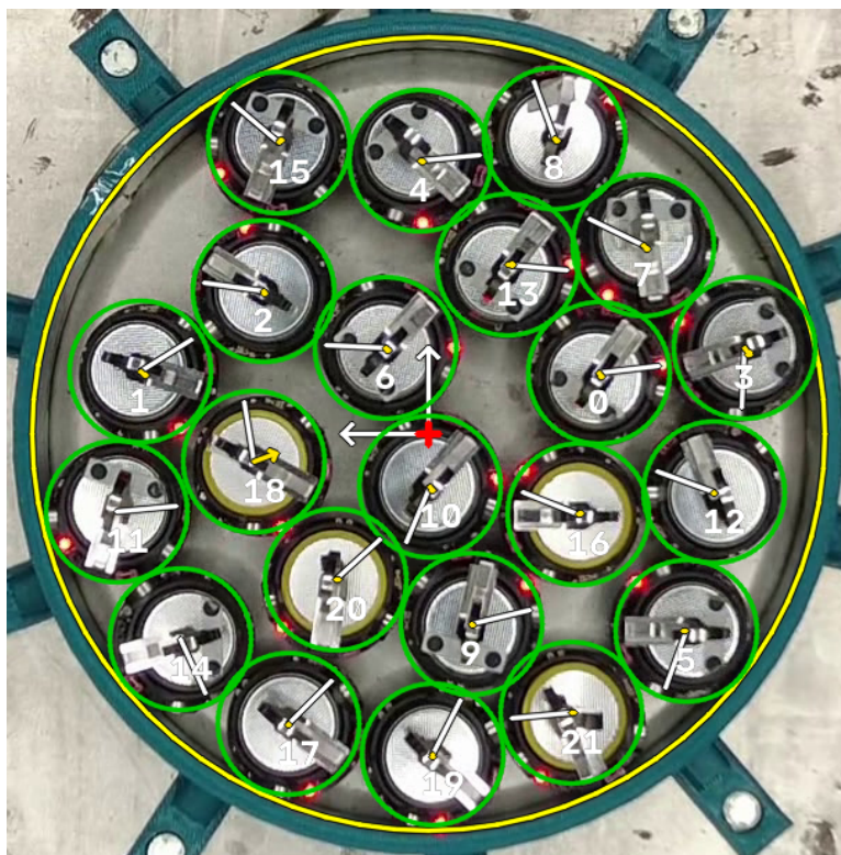
Figura 15: Cuadro de ejemplo con identificador, vector velocidad (amarillo, largo = desplazamiento en 7,5 cuadros) y orientación (aguja blanca). Círculo verde: posición observada; naranja: estimada. Imagen tal como la graba la cámara (espejada); flecha y aguja dibujadas sobre ella.
