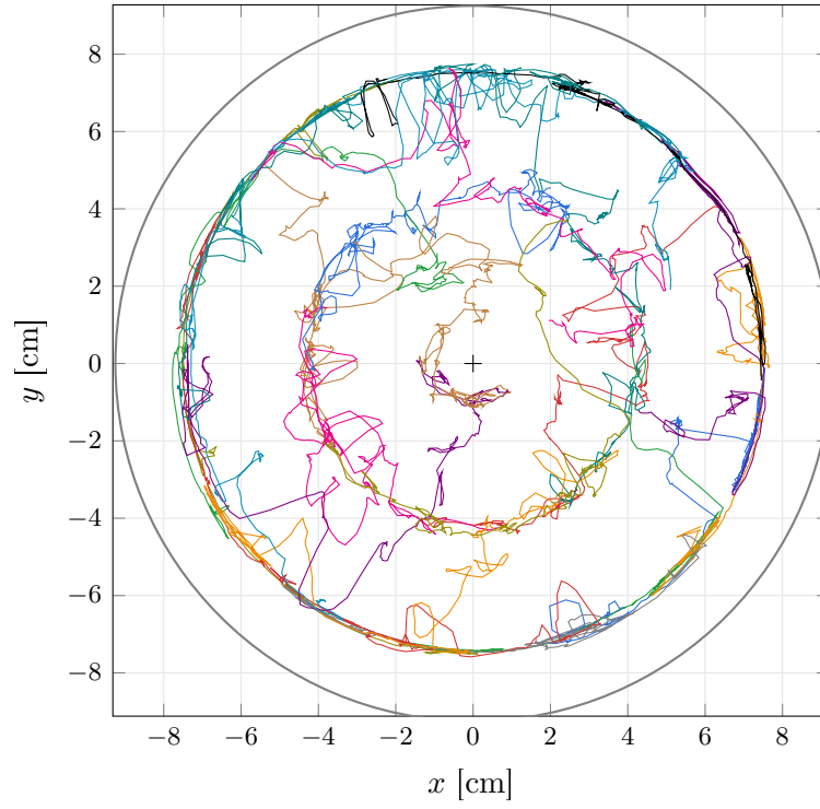
Figura 13: Trayectorias de los 22 robots (escena real, video espejado corregido; origen en el centro del recinto, y hacia arriba; círculo gris: pared interior), primeros 5 minutos reales.
