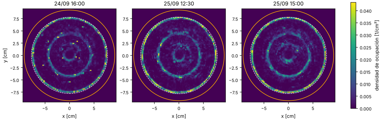
Figura 6: Densidad de ocupación de los centros de los robots durante todo cada ensayo, con origen en el centro del recinto de cada cuadro ( y hacia arriba, escena real). Círculo naranja: pared interior ( R_{\text{int}} ); punteado blanco: radio de contacto R_c (percentil 99,5 de r , centros de los robots apoyados en la pared).
