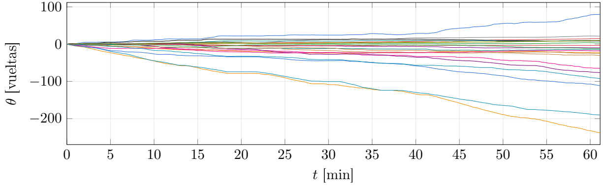
Figura 24: Orientación acumulada de cada robot ( \theta = 0 en el primer cuadro; positivo = antihorario).
