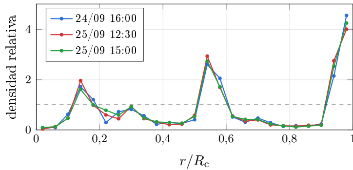
Figura 7: Densidad radial de los centros normalizada por área (1 = distribución uniforme); R_c es el radio máximo que alcanzan los centros.
