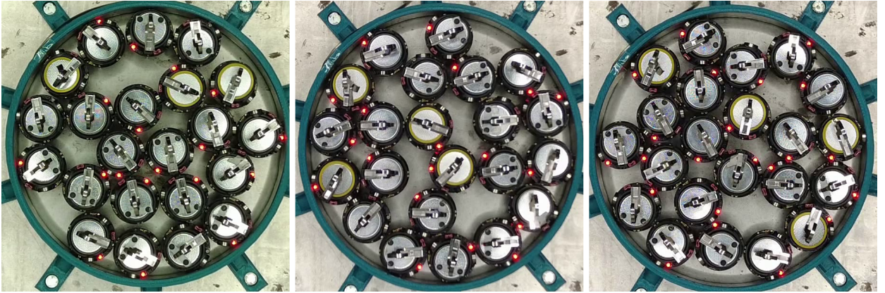
Figura 9: Un cuadro durante el atasco principal de cada ensayo (de izquierda a derecha: 24/09 16:00, minuto 47,8; 25/09 12:30, minuto 50,6; 25/09 15:00, minuto 19,7). Imágenes tal como las graba la cámara (espejadas). Los robots siguen encendidos (LEDs rojos), pero durante el atasco prácticamente no se desplazan ni giran.
