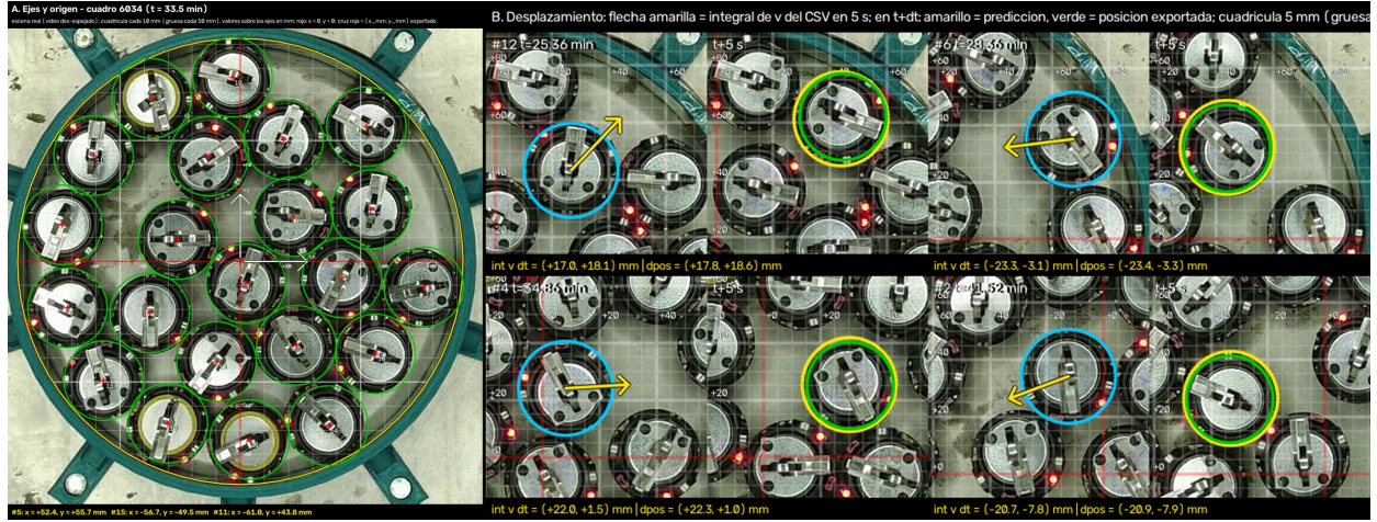
Figura 2: Verificación de 24/09 16:00. Izquierda: cuadro des-espejado con los robots redibujados solo con (x, y) del CSV (cruz roja), el recinto (amarillo), los ejes y una cuadrícula de 10 mm en el sistema del recinto (valores sobre los ejes). Derecha: cuatro robots en t (celeste: posición; flecha: integral de la velocidad en 5 s) y en t + 5s (amarillo: predicción; verde: posición exportada), sobre una cuadrícula de 5 mm.
