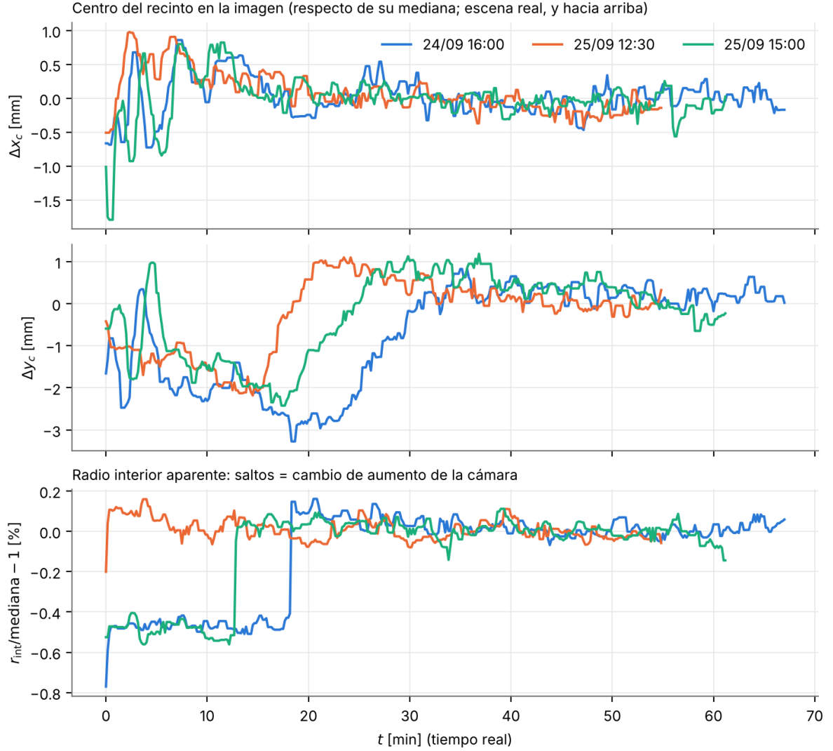
Figura 1: Centro del recinto (respecto de su mediana, escena real) y radio aparente a lo largo de cada ensayo, después de la mediana móvil de 5 muestras. Los saltos del radio coinciden con un agrandamiento igual de la placa de fondo: son cambios de aumento de la cámara.
