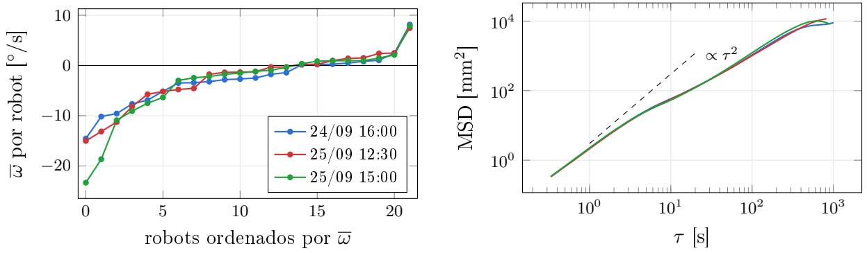
Figura 6: Izq.: velocidad angular media de cada robot, ordenada (cada punto es un robot). Der.: desplazamiento cuadrático medio \text{MSD}(\tau) = \langle |\vec{r}(t + \tau) - \vec{r}(t)|^2 \rangle ; la recta de referencia indica movimiento balístico.
