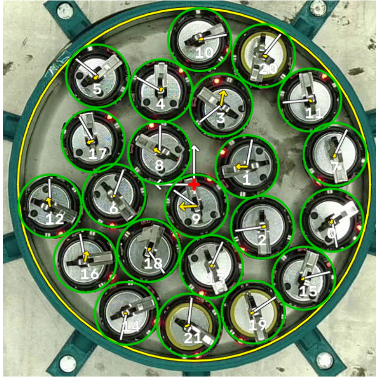
Figura 11: Cuadro de ejemplo con identificador, vector velocidad (amarillo, largo = desplazamiento en 7,5 cuadros) y orientación (aguja blanca). Círculo verde: posición observada; naranja: estimada. Imagen tal como la graba la cámara (espejada); flecha y aguja dibujadas sobre ella.
