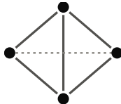
K_4 - e \rho = 2.5083
